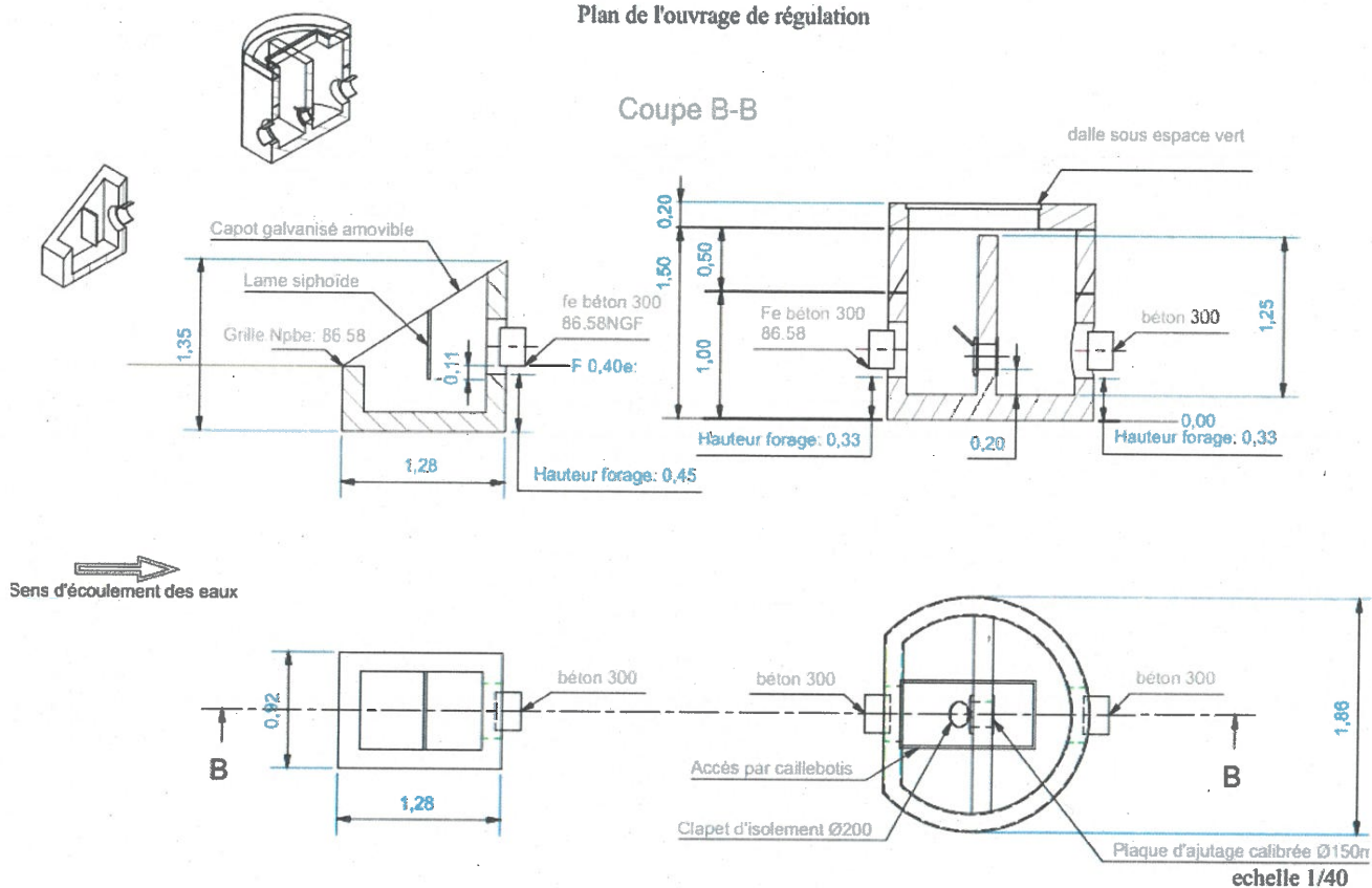
Plan de l'ouvrage de régulation
