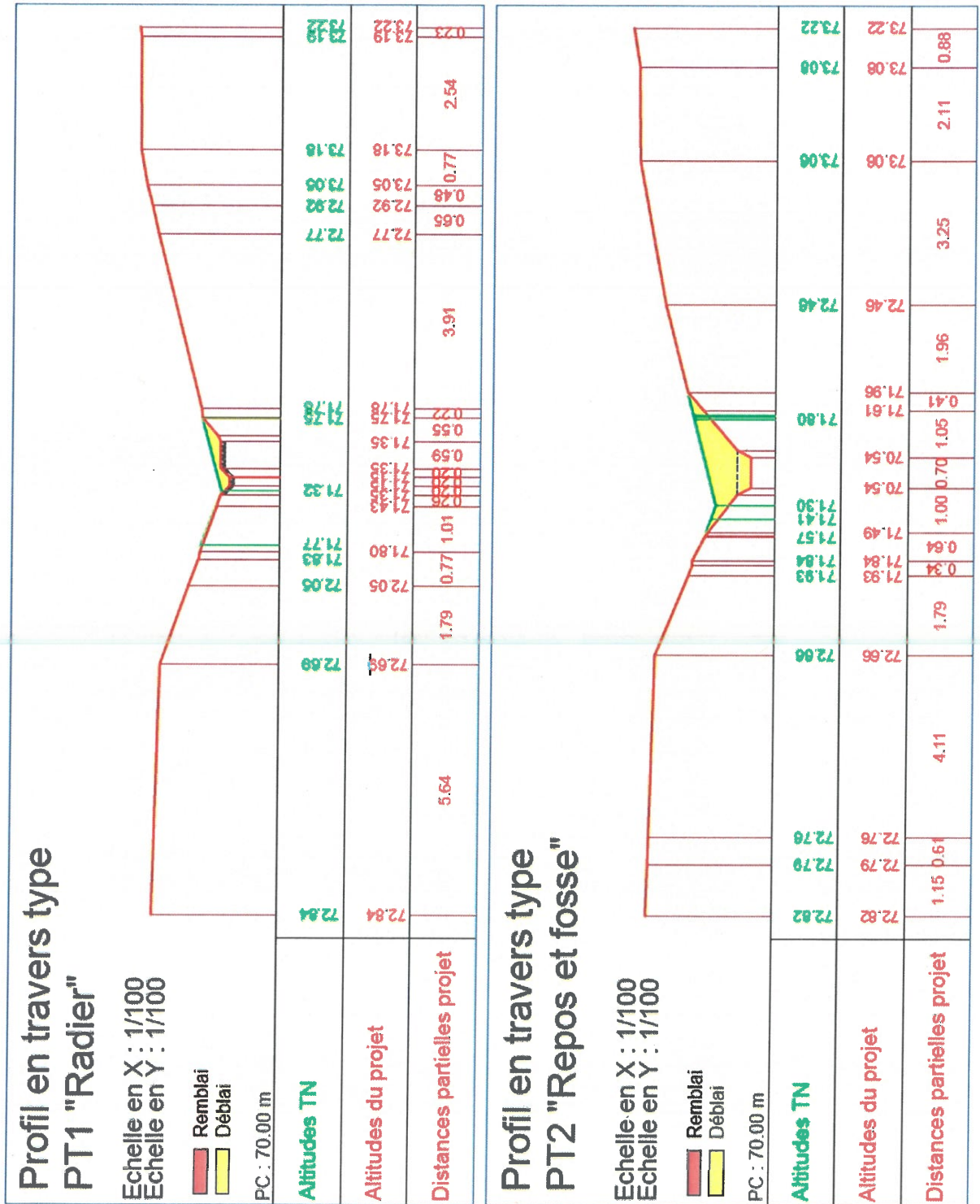
Annexe 5 : Profils en travers type au droit des radiers et fosses
